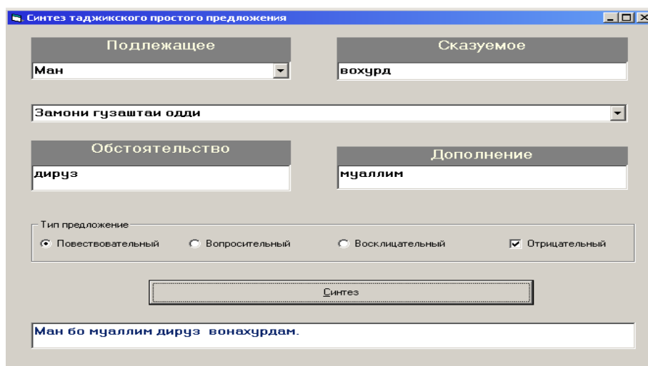
Рас. 2. Натиҷаи кори барномаи синтези ҶСТ
